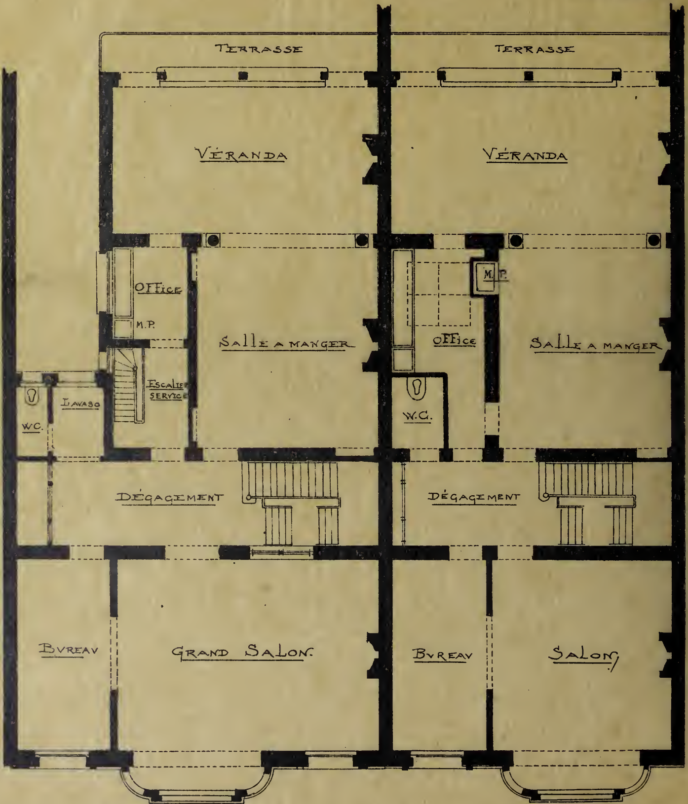
PLAN DU BEL-ETAGE.
